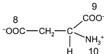
aspartate
